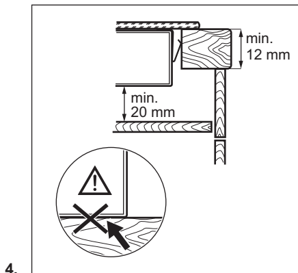
4. INSTALLAZIONE INTEGRATA
